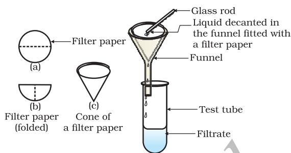
Fig. 2.2: Filtration
